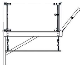
DÉTAIL W ECHELLE 1 : 5
