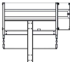
DÉTAIL Y ECHELLE 1 : 5
